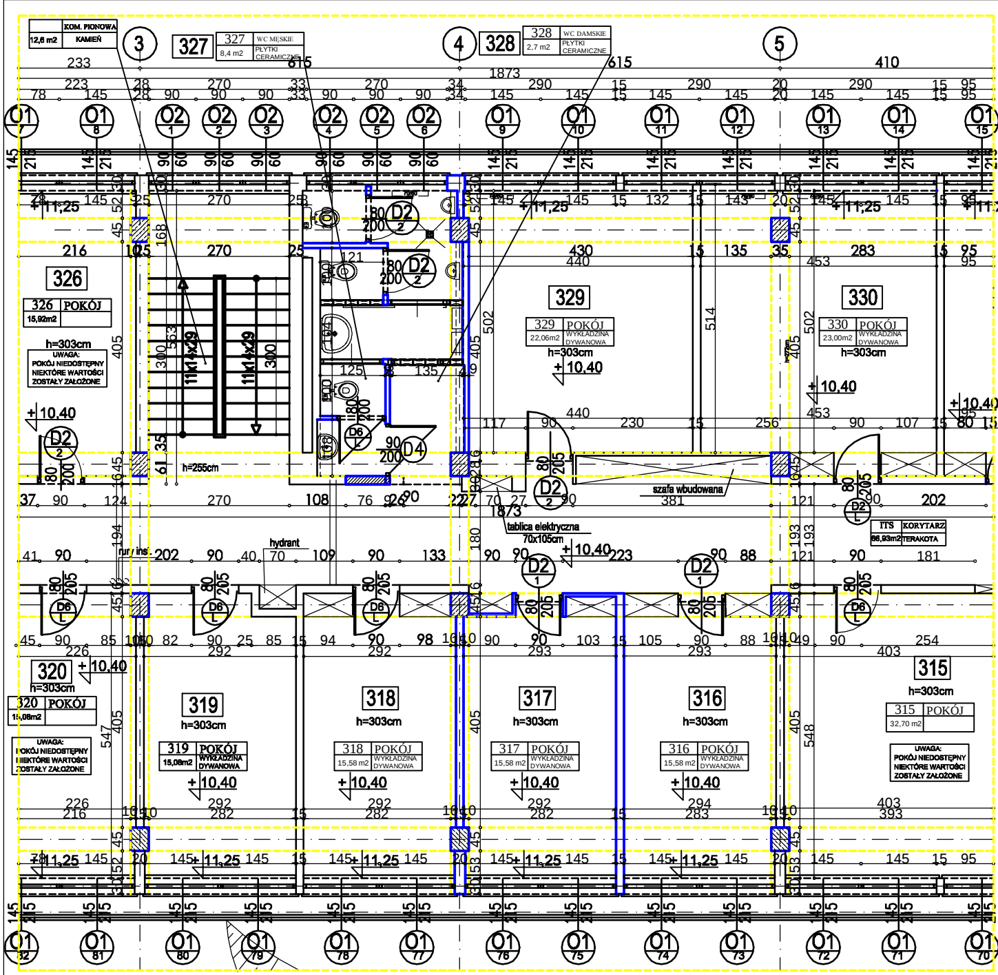
RZUT NA POZIOMIE +200 CM NAD POSADZKĄ
